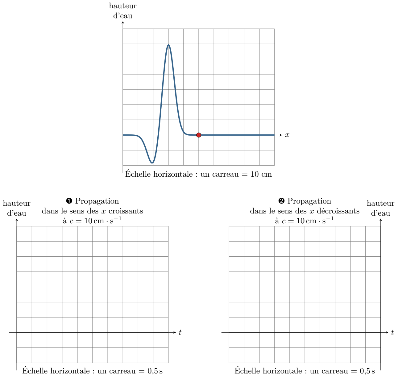
Figure 1 – Représentations d’une onde plane progressive.
