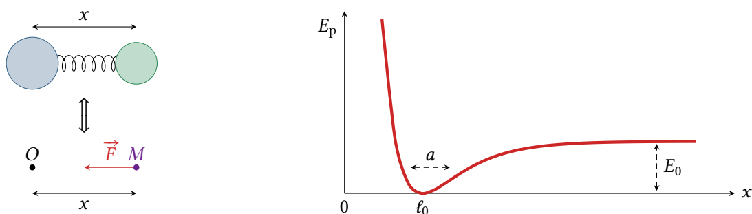
Figure 3 – Modélisation d'une molécule diatomique.
