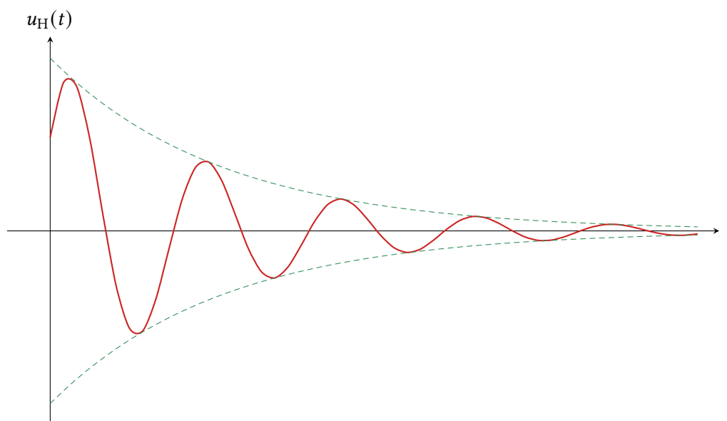
Figure 4 – Exemple d'allure de la solution homogène en régime pseudo-périodique.
