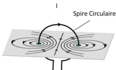
(b) Spire circulaire plane (vue 3d)
